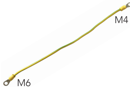
1x „Erdungsleiter 2“ mit Ringösen M6 - M4 (0,2m)
